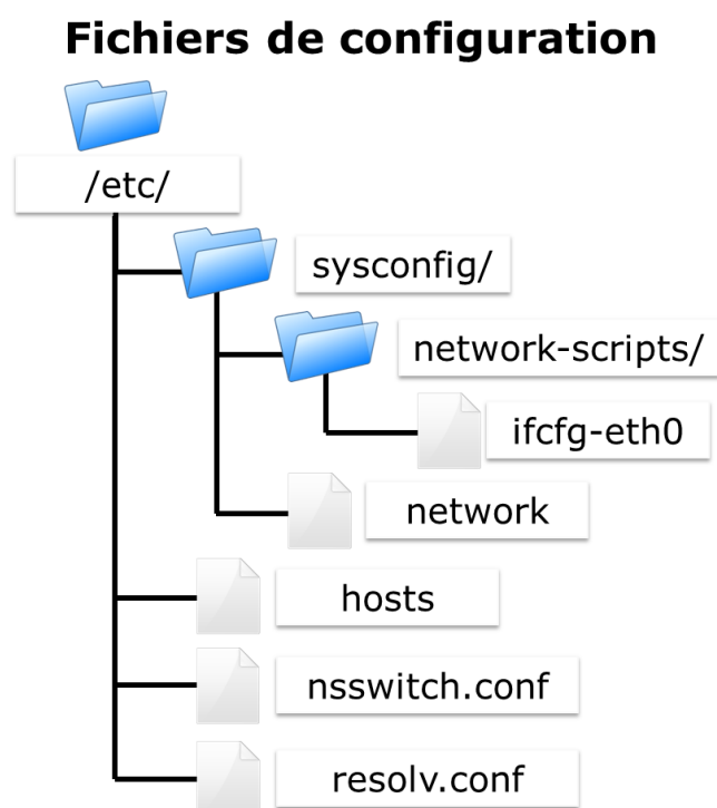
Figure 34. Synthèse des fichiers mis en oeuvre dans la partie réseau
