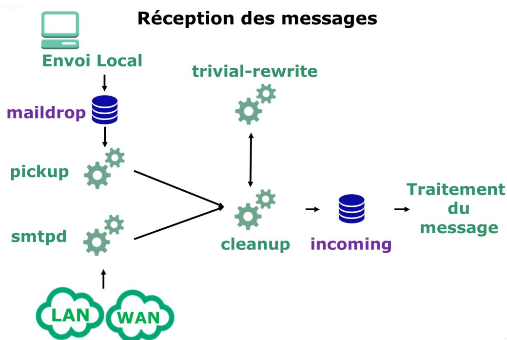
Figure 59. Synoptique de postfix partie réception des messages
