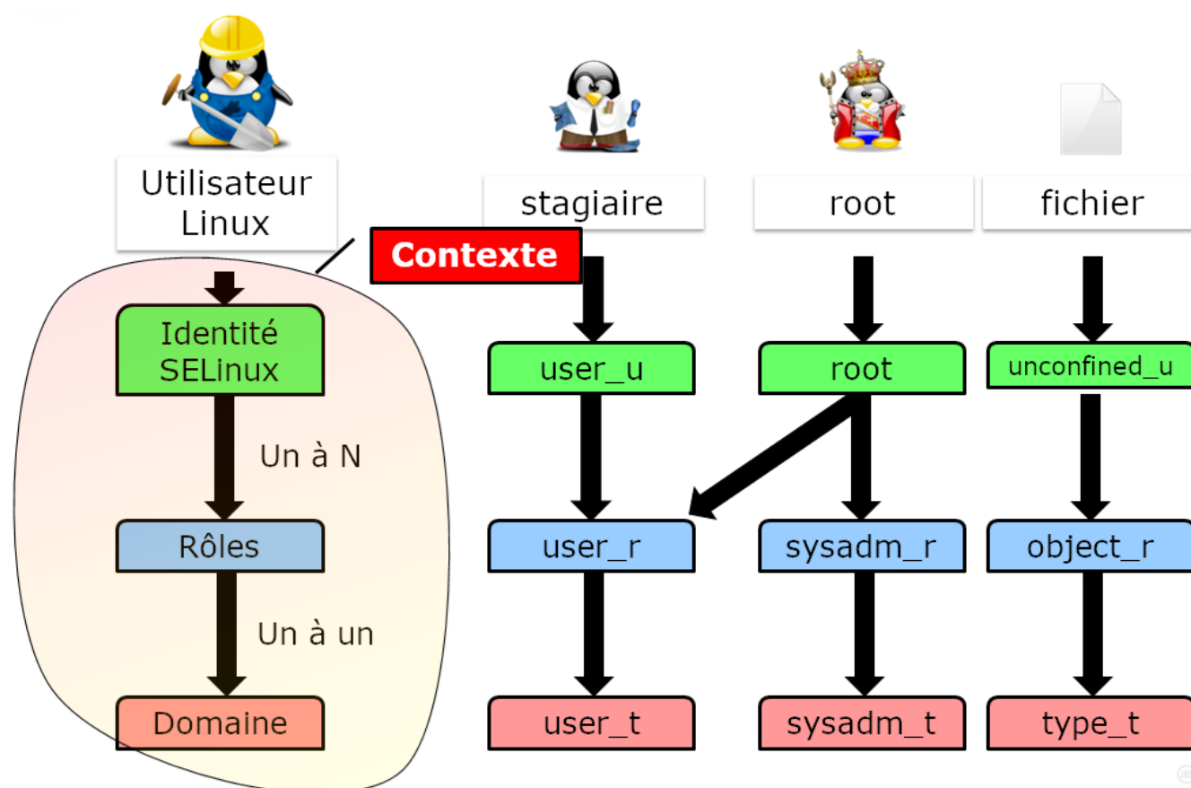
Figure 37. Le contexte SELinux
