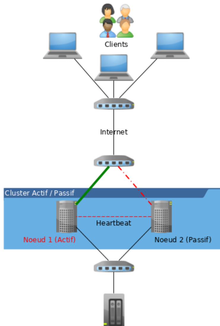
Figure 71. Schéma d'un cluster actif/passif
