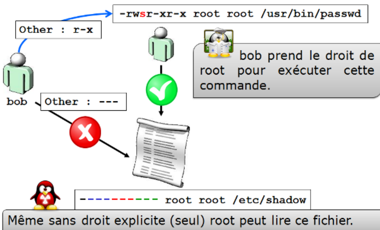
Figure 25. Fonctionnement du SUID
