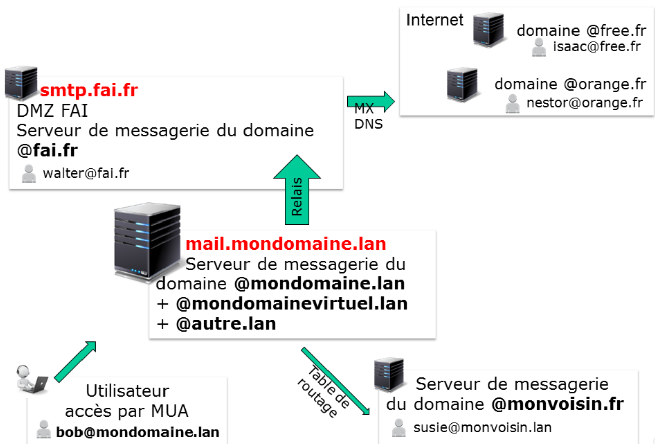
Figure 56. Synoptique global du système de messagerie
