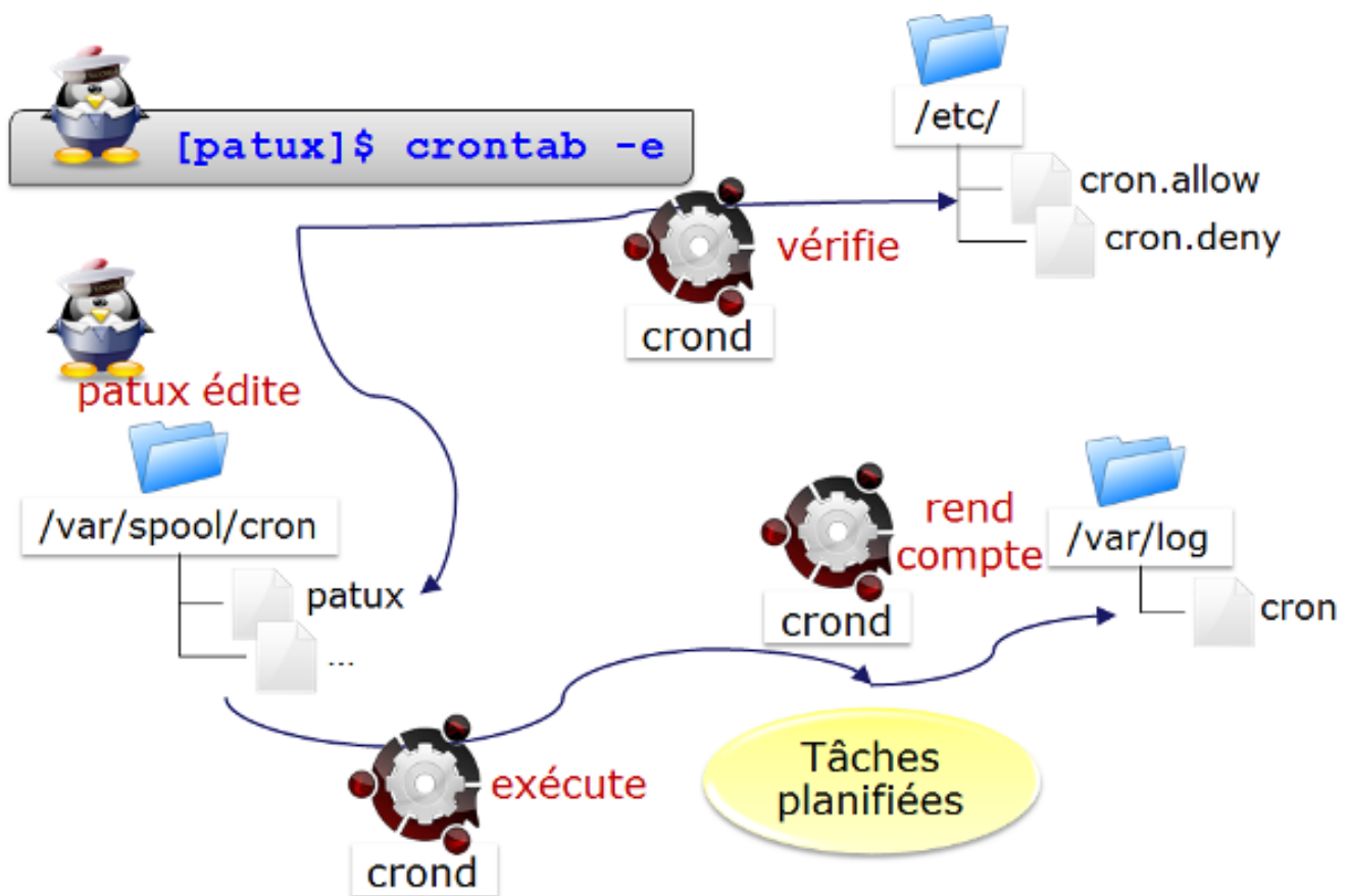
Figure 31. Processus d'exécution d'une tâche
