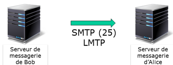
Figure 51. Le transfert de message entre MTA
