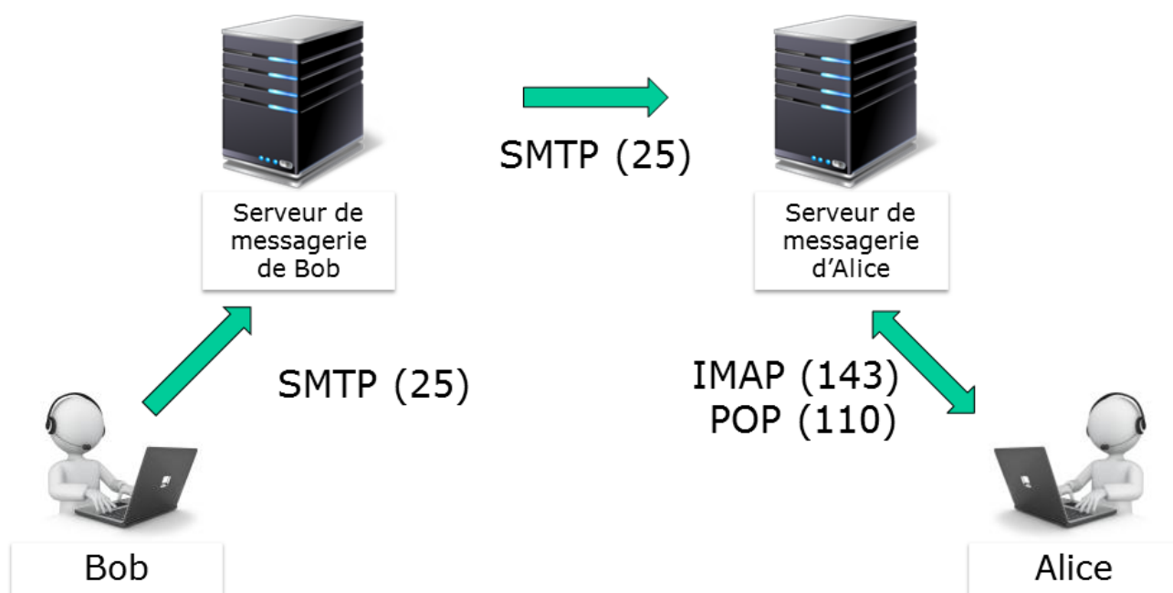
Figure 50. Les protocoles de messagerie mis en oeuvre
