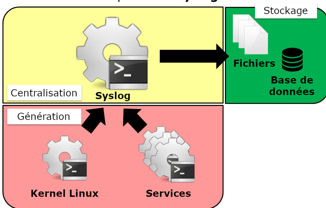
Figure 62. Fonctionnement du protocole Syslog
