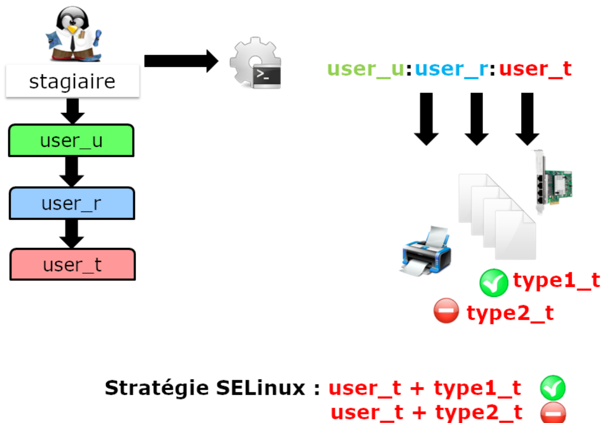
Figure 38. Le contexte SELinux d'un processus standard
