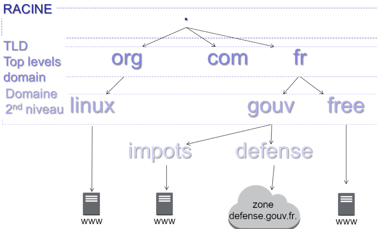
Figure 40. Principe de fonctionnement du DNS
