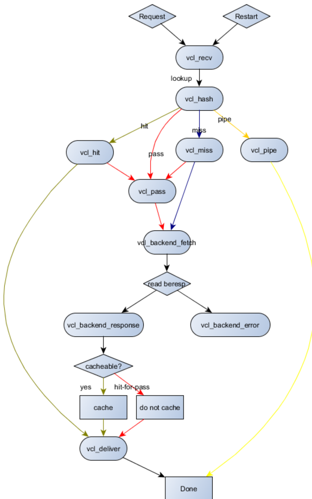
Figure 70. Fonctionnement simplifié de varnish
