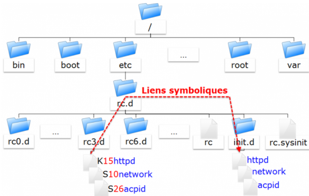
Figure 29. Synthèse de l'arborescence système liée au démarrage
