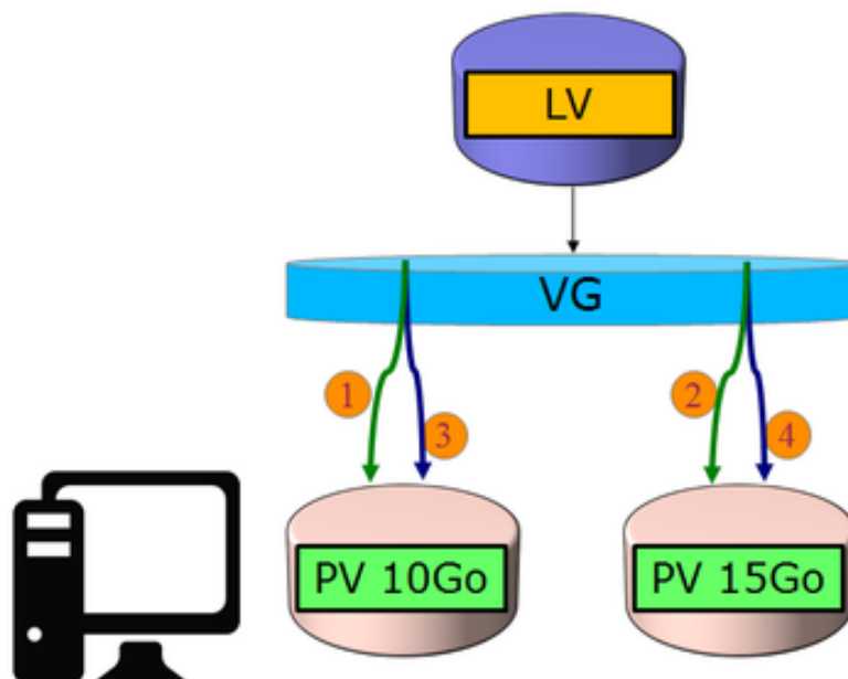
Figure 15. Volumes en mode stripe
