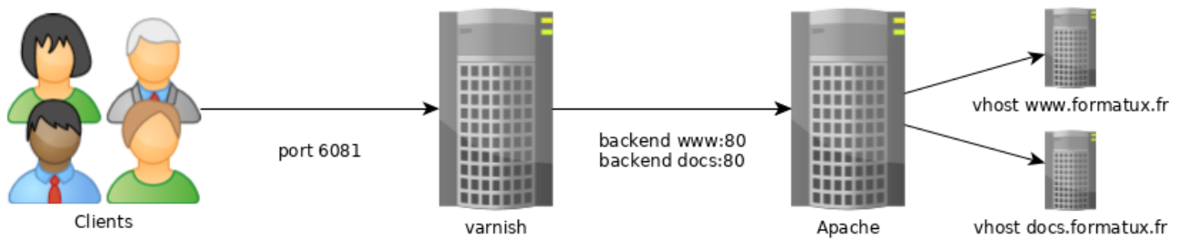
Figure 67. Fonctionnement par défaut de Varnish
