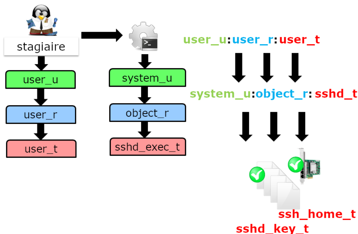
Figure 39. Le contexte SELinux d'un processus important - exemple de sshd
