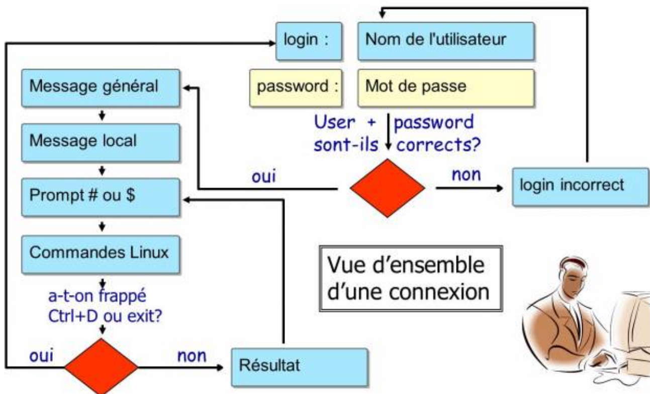
Figure 7. Principe de fonctionnement du SHELL
