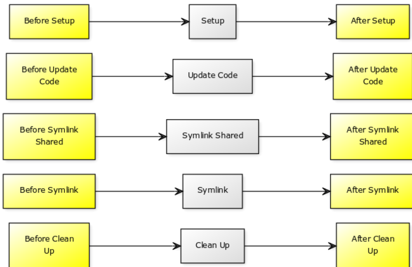
Figure 78. Etapes d'un déploiement
