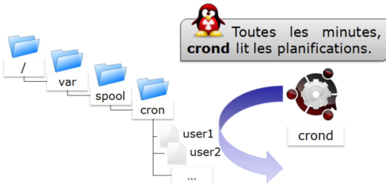
Figure 30. Arborescence de cron
