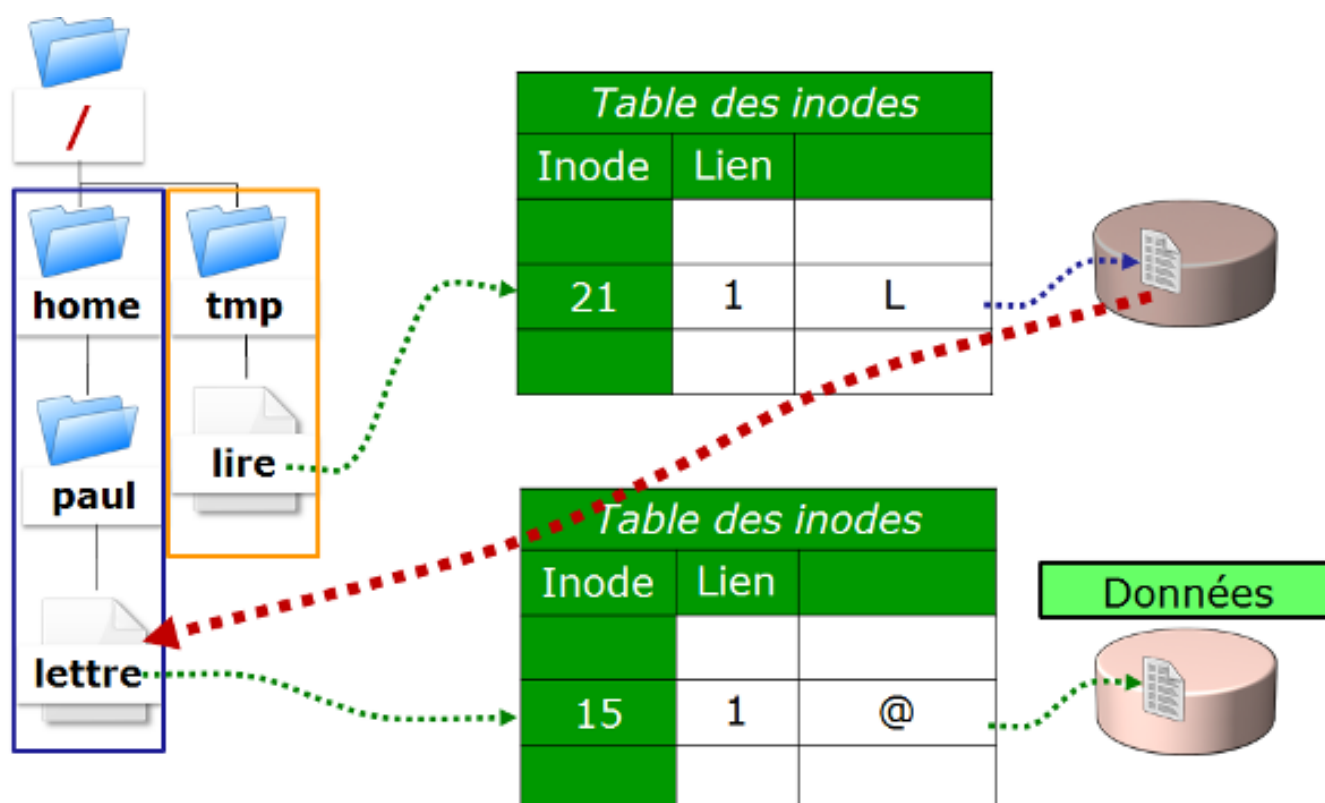
Figure 19. Représentation d'un lien symbolique
