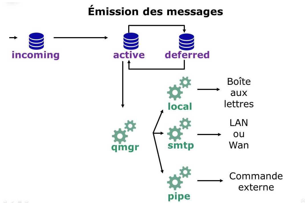
Figure 60. Synoptique de postfix partie émission des messages
