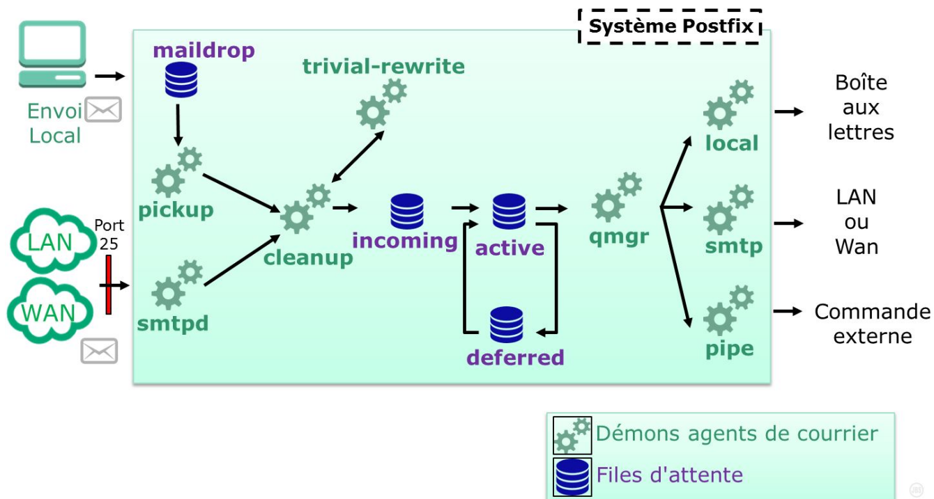
Figure 58. Synoptique global de postfix
