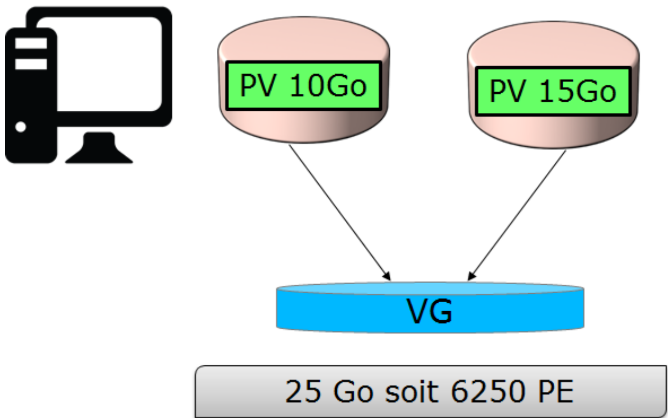
Figure 13. Groupe de volumes, taille de PE égale à 4Mo
