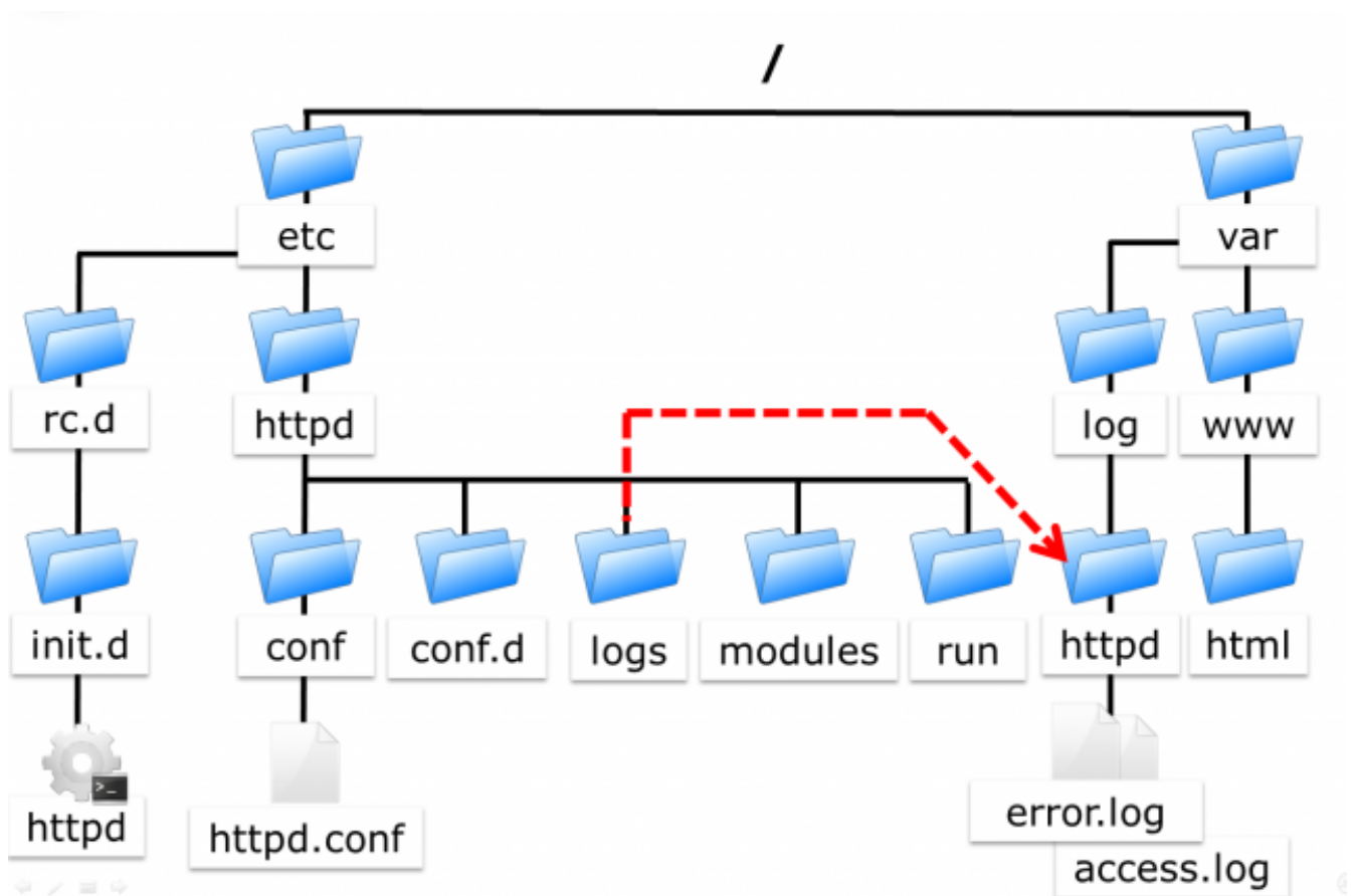
Figure 44. Arborescence d’Apache
